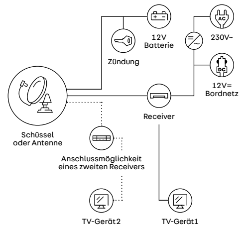
→ Vereinfachtes Anschlussschema
